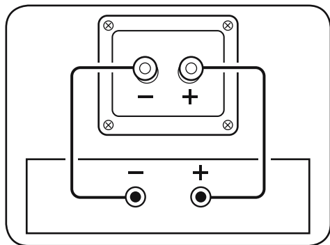
Standardtilkopling
